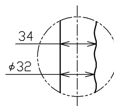
握りバー形状詳細（1:3）
